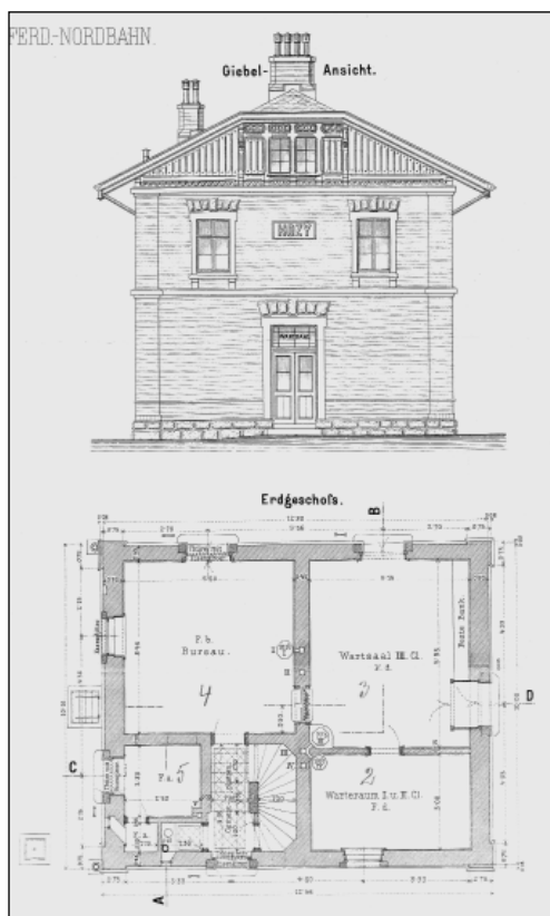
Typový plán výpravní budovy IV. třídy, r. 1886, České dráhy a.s. – GR 04, depozitář v Července
